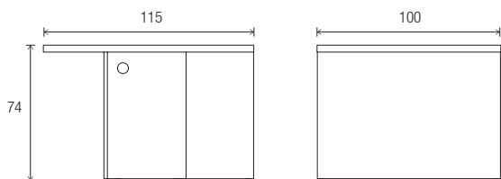
Low DDA module***
